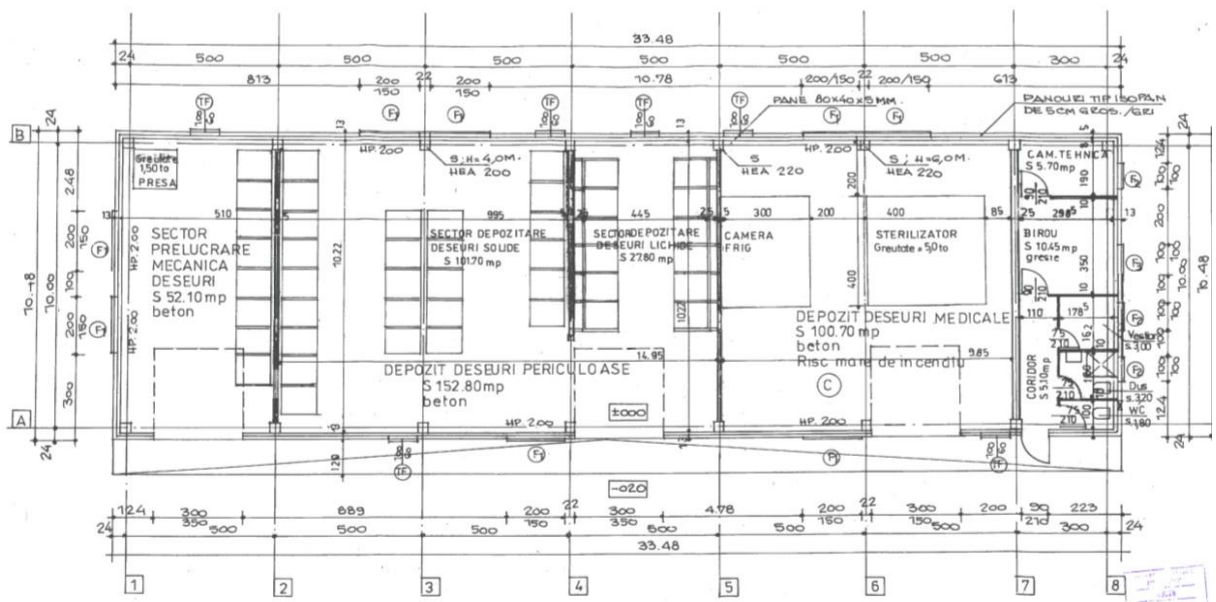
Fig.1. Repartizare hală
