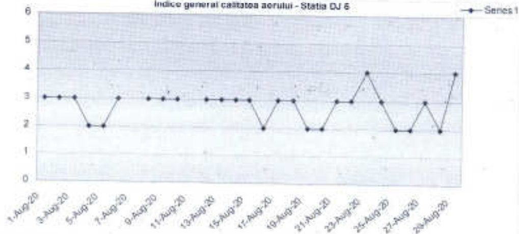
Indice general calitatea aerului - Statia DJ 6
