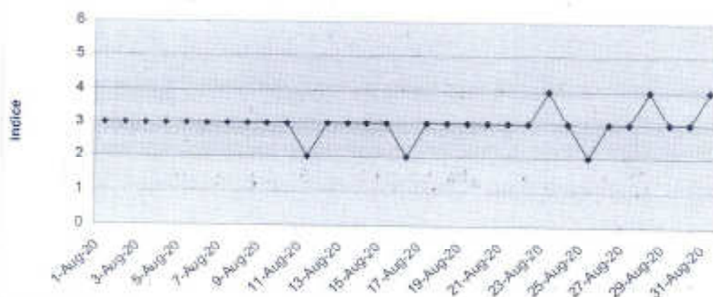
Indice general calitatea aerului- statia DJ5
