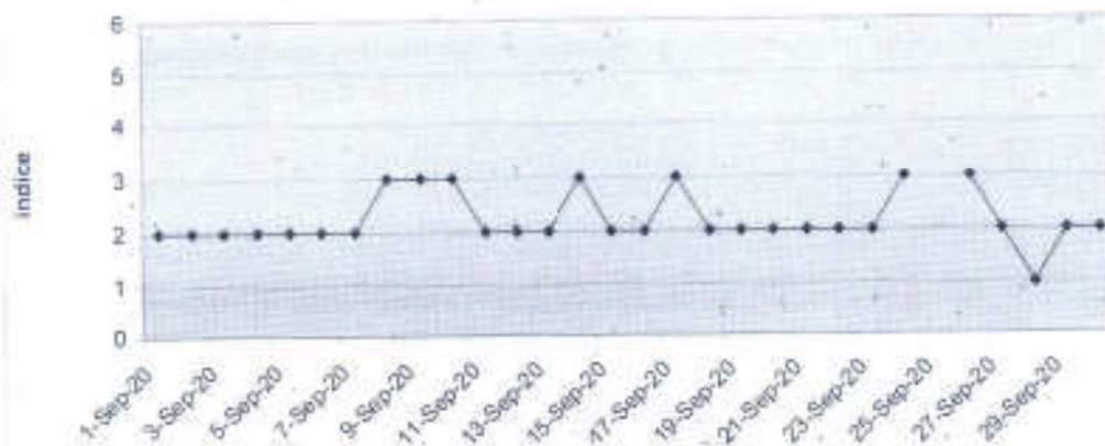
Indice general calitate a aerului- statia DJ1
