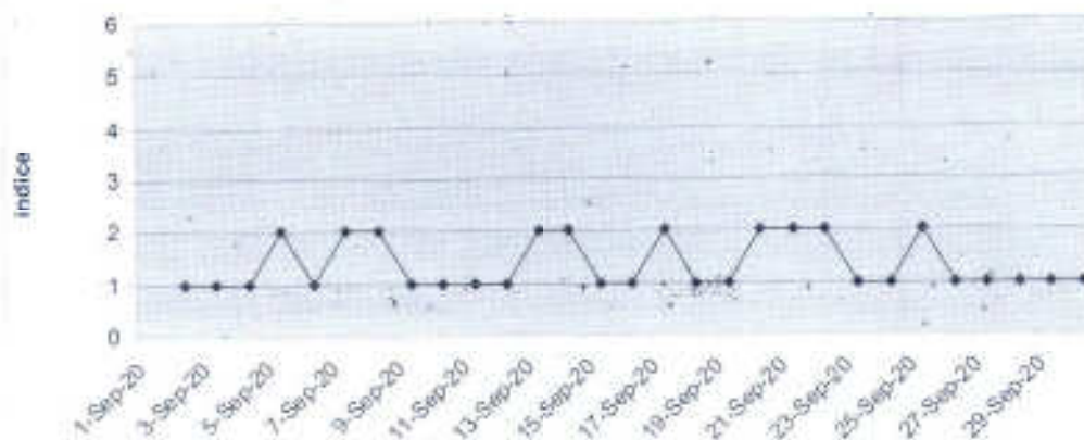
Indice general calitate a aerului - statia DJ2
