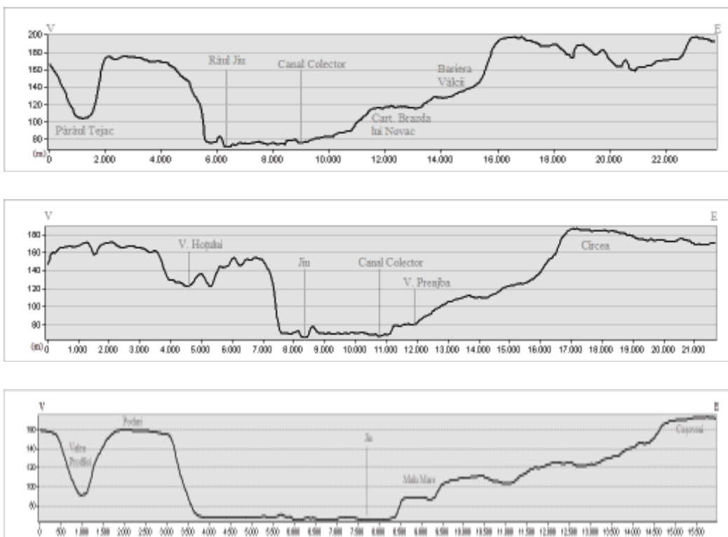
Figura 2-8 Succesiune de profile transversale
